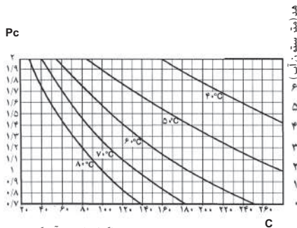
دیگرام ظرفیت آب گیری
